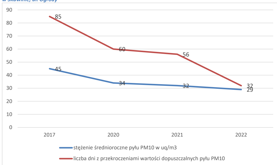
Wykres 26. Stężenia średnioroczne [ \mu\text{g}/\text{m}^3 ] w przedziale czasowym 2017-2022 mierzone na stacji pomiarowej w Skawinie, ul. Ogrody
